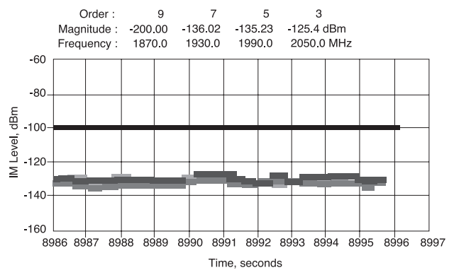
REVERSE IM N Type Connector Data
