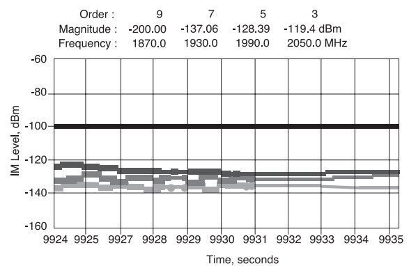
REVERSE IM SMA Connector Data
