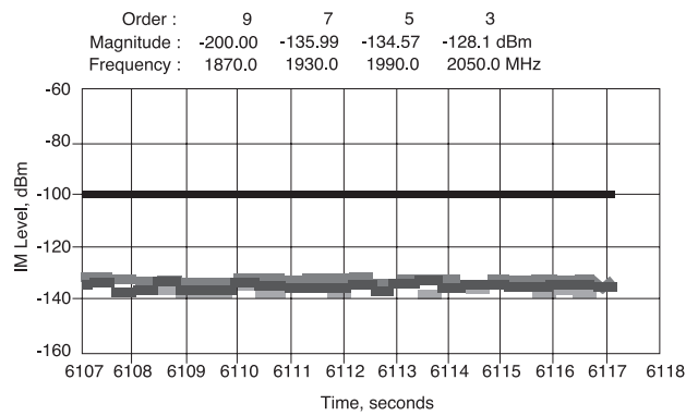
REVERSE IM 7/16 Connector Data
